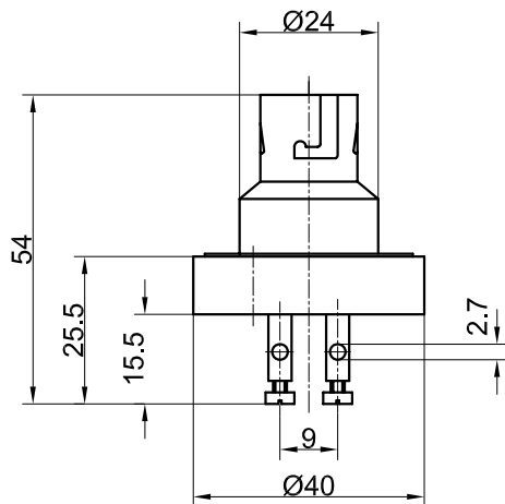
Bajonett-Fassung BA 15d / B 15d
