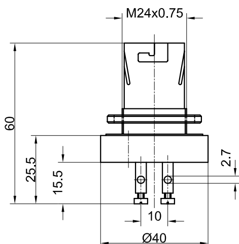
Bajonett-Fassung BA 20d / B 20d mit Gewinde
