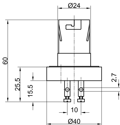
Bajonett-Fassung BA 20d / B 20d normal
