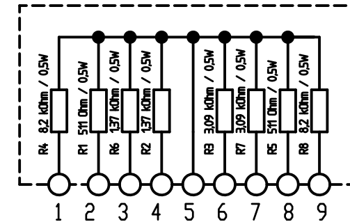
Innenschaltung
