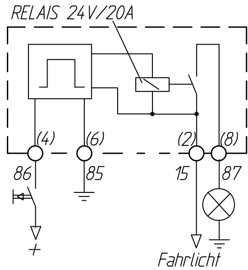
Prinzipschaltbild
