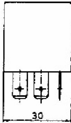
Steckeranordnung Terminal Layout
