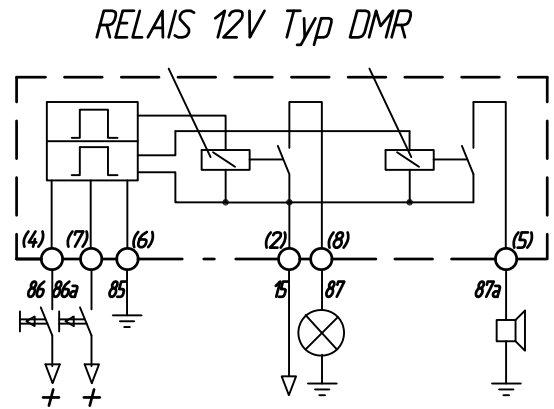
Prinzipschaltbild
