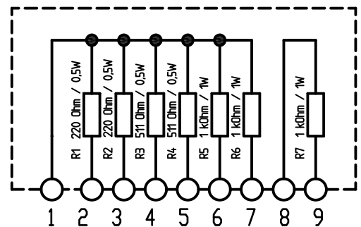
Innenschaltung
