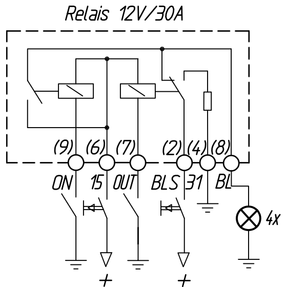
Prinzipschaltbild
